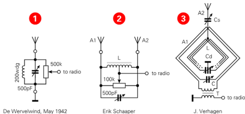
Hierboven worden schema's van drie versies voor een Moffenzeef getoond
